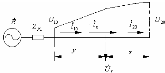
图3 无补偿空载线路
