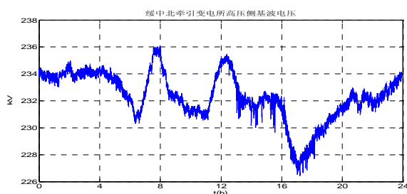
图 2 绥中北牵引变电所高压侧基波电压
