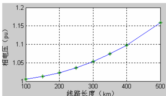
图 4 线路末端电压
